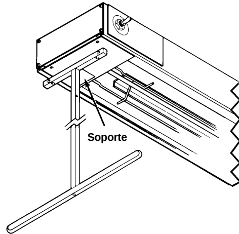
Figura 5. Montaje alternativo de pata en T
