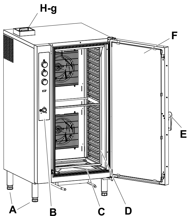
GASMODELL 20 GN 1/1
