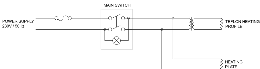
FIG. n°5 - Schema elettrico del Dispenser
