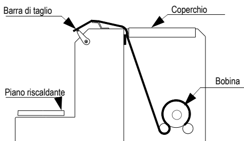
FIG. n°7 - Caricamento del vitafilm
