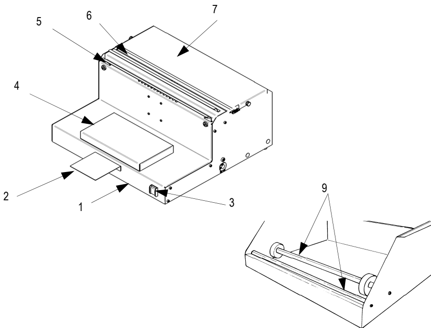
FIG. n°1 - Veduta generale della macchina
