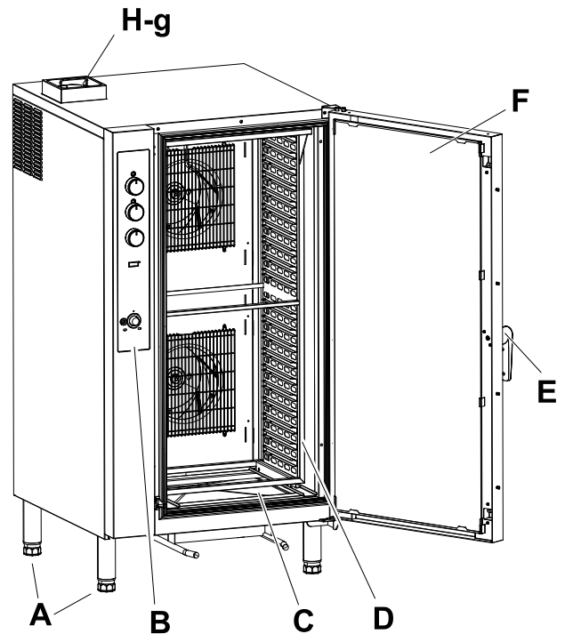
Modelos de GAS 20 GN 1/1
