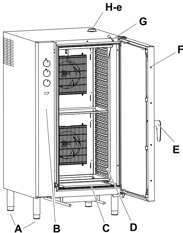
Modelo ELÉCTRICO 20 GN 1/1
