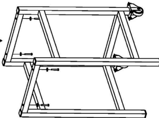
MONTAGGIO CAVALLETTO
