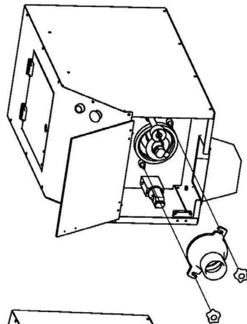
MONTAGGIO CONO
