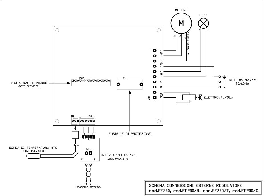
Fig. 3: Schéma des connexions externes du variateur.
