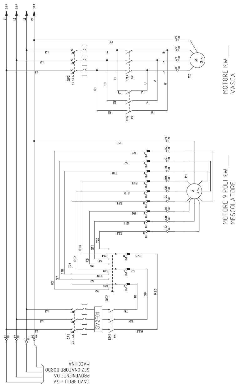
FIG. / РИС. 16 - MX40/60/80 TV Schema elettrico / Electrical diagram / Schemas electriques / Diagrama eléctricos / Монтажная схема
