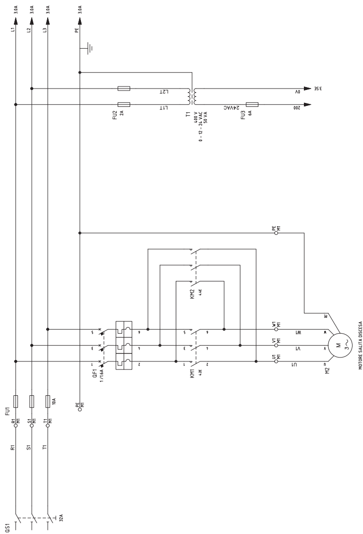
FIG. / PИC. 22 - MX40/60/80 PV Schema elettrico / Electrical diagram / Diagrama electric / Schemas electriques / Diagrama eléctricos / Montajная схема
