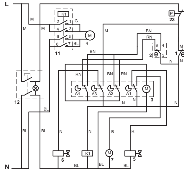
VERSIONE AD ACQUA / WATER COOLED / VERSION AGUA
