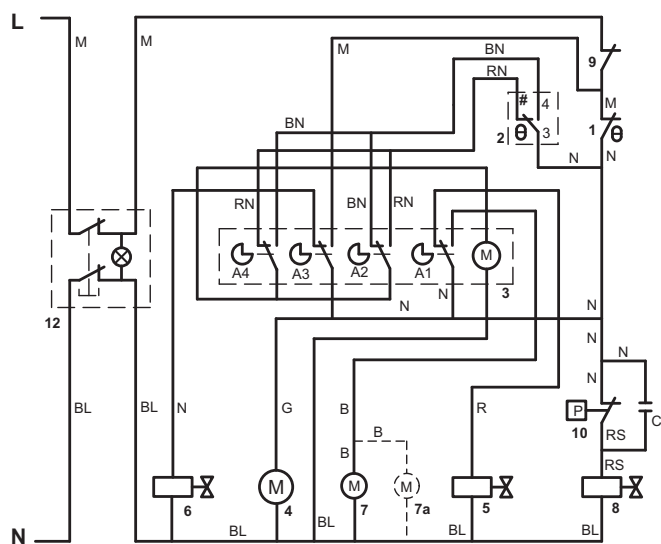
VERSIONE AD ACQUA / WATER COOLED / VERSION AGUA
