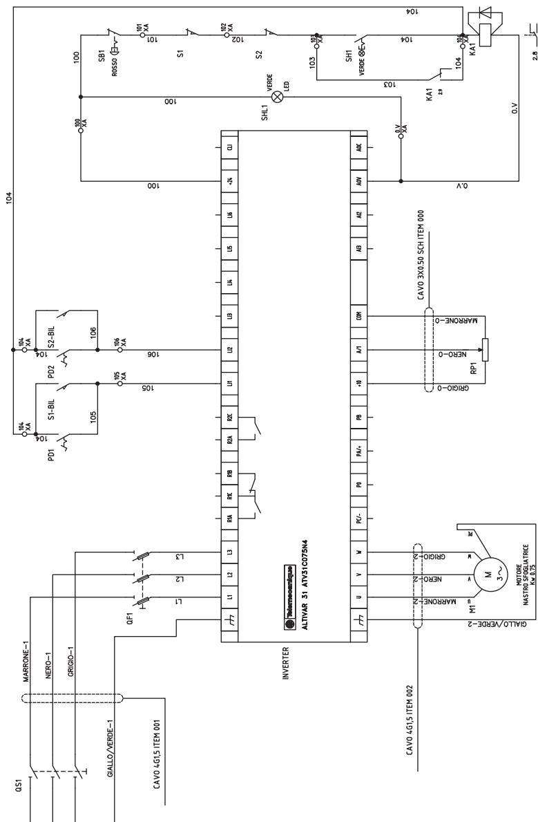
FIG. / ABB. / РИС. / ПИС. 19 - SF600P-ST500P Schema elettrico / Electrical diagram / Schemas electriques / Diagramas eléctricos Elektroschaltpläne / Электрические схемы
