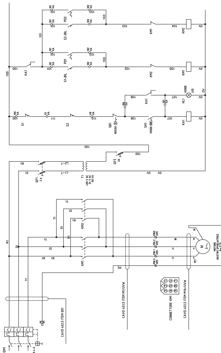
FIG. / ABB. / РИС. 18 - SF600 Schema elettrico / Electrical diagram / Schemas electriques / Diagramas eléctricos Elektroschaltpläne / Электрические схемы
